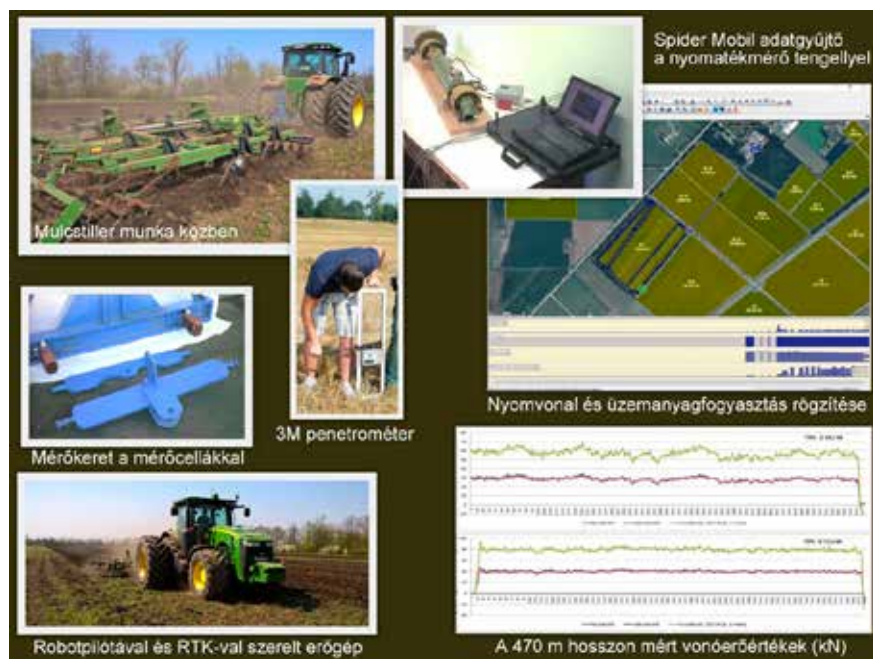
2. ábra: A jelenlegi eszközpark (Karcag, 2017), Forrás: CZIMBALMOS ET AL. (2017)
