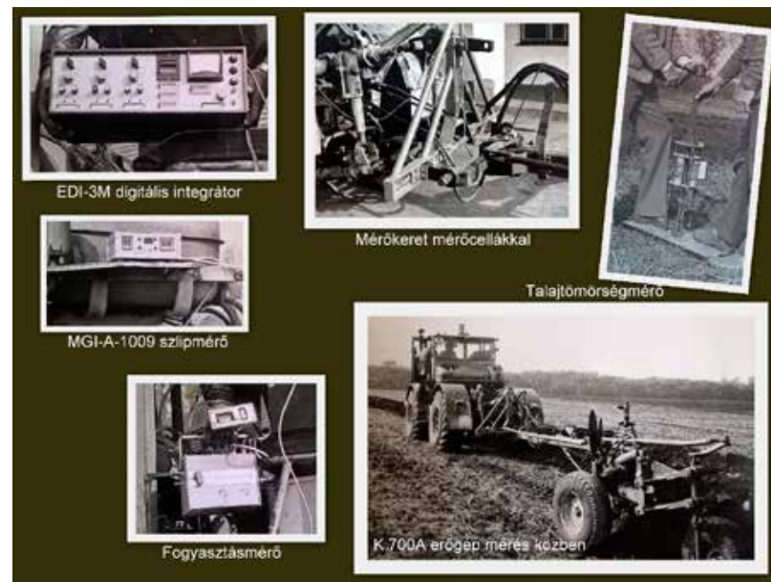
1. ábra: A korabeli mérőeszközpark (Karcag, 1982), Forrás: KAPOCSI ET AL. (1982)
